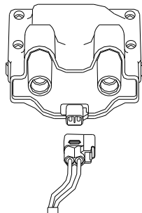
図⑤ No.9535-70用 スズキ2端子閉磁路／但し同時点火車、ダイレクト点火車を除く
