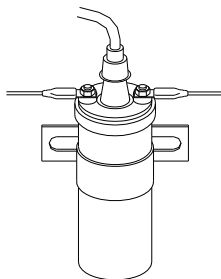
図⑥ No.9529-10用 円筒形コイル(三菱車、マツダ車及びポイント点火の車輛を除く)
