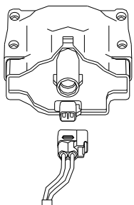
図③ No.9521-10用 デンソー2端子閉磁路／但し同時点火車を除く
